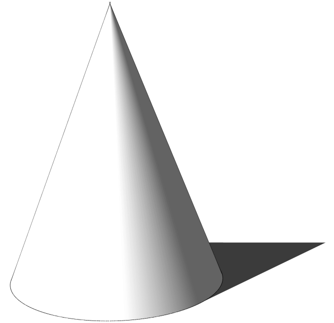
un cône
