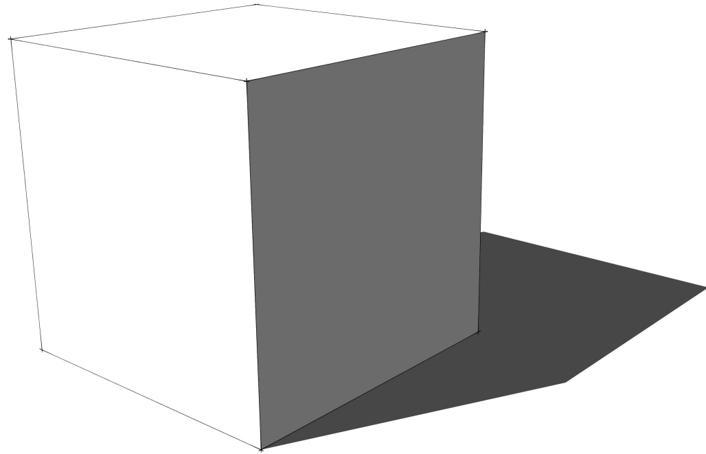
un cube
