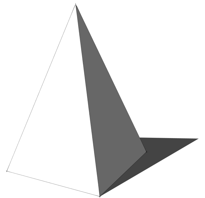
une pyramide
