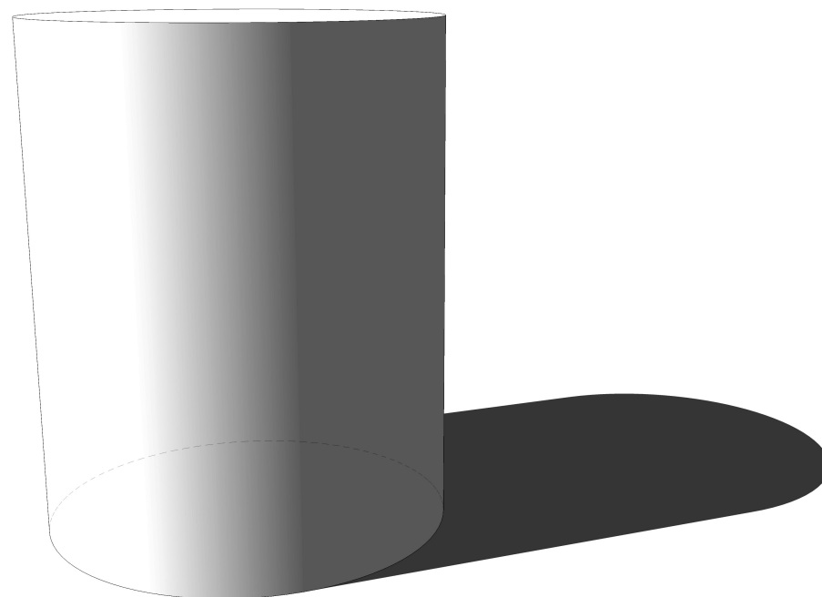
un cylindre
