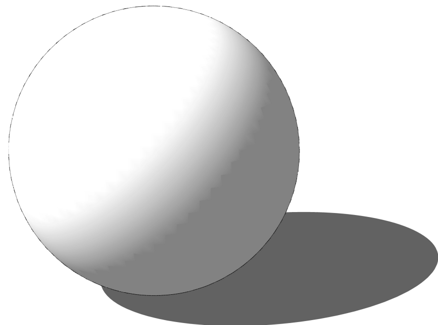
une sphère
